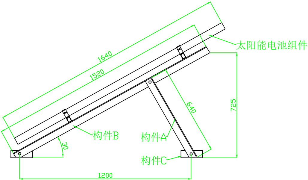
支架整体安装侧视图
