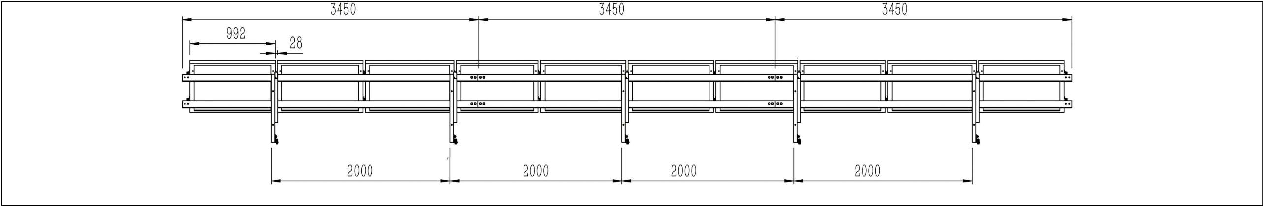
支架整体安装主视
